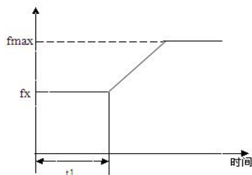
图 F1-1 起动频率示意图
