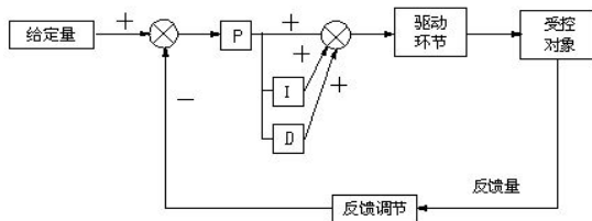
图 F7-2 PID 调节示意图
