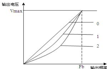
图 F2-1 V/F 曲线示意图
