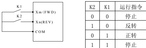
图 F5-1 二线式控制模式 1 示意图
