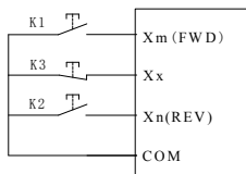
图 F5-3 三线式控制模式 1 示意图
