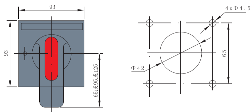
方形手柄外形及开孔尺寸
