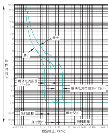
TGM1L-225(配电保护用)
