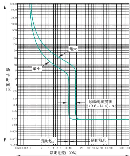
TGM1L-800(电动机保护用)
