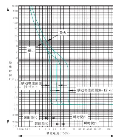
TGM1L-400(配电保护用)
