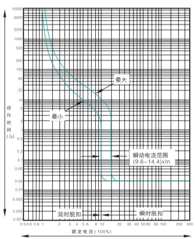
TGM1L-225(电动机保护用)
