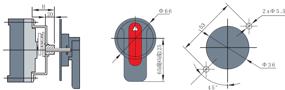
手柄操作机构
