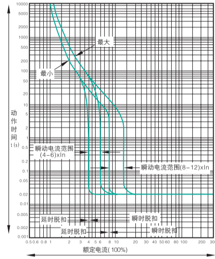
TGM1L-800(配电保护用)
