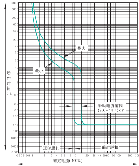
TGM1L-400(电动机保护用)
