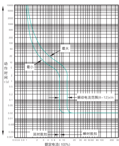
TGM1L-100(配电保护用)
